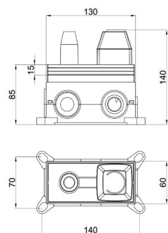
مکانیزم دوش توکار ونوس و مارس
