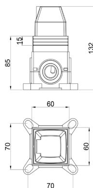
مکانیزم توالت و روشویی توکار ونوس و مارس
